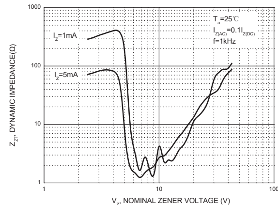
Fig. 6 Effect of Zener Voltage on Zener Impedance
