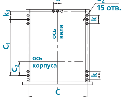
Расположение отверстий крепления вентиляторов
