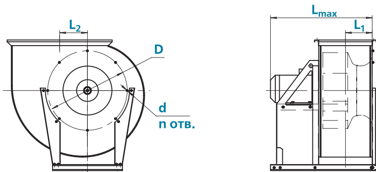
Выходной фланец вентиляторов
